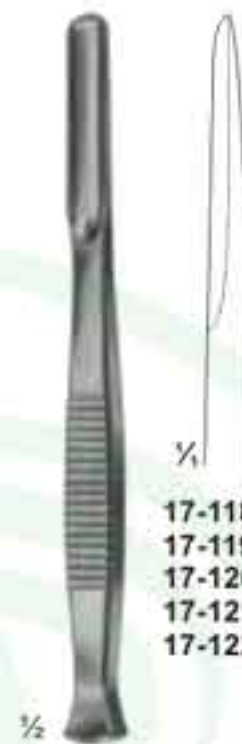
17-118 - 122 Gouges 140 mm
